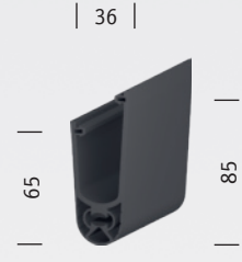
SENTIR edge 65/85 ST 1509-0920
